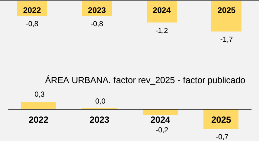
TOTAL PAÍS. factor rev_2025 - factor publicado
