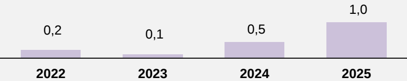
Área Urbana. Método ajustado - método anterior
