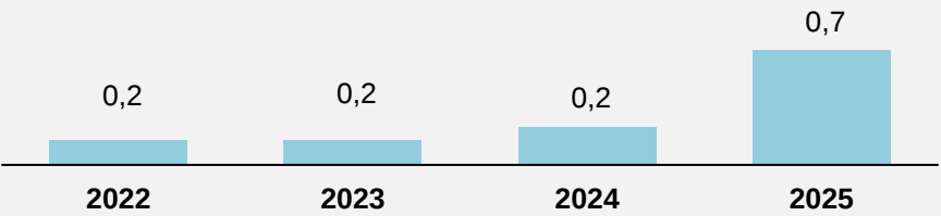
Área Urbana. Método ajustado - método anterior
