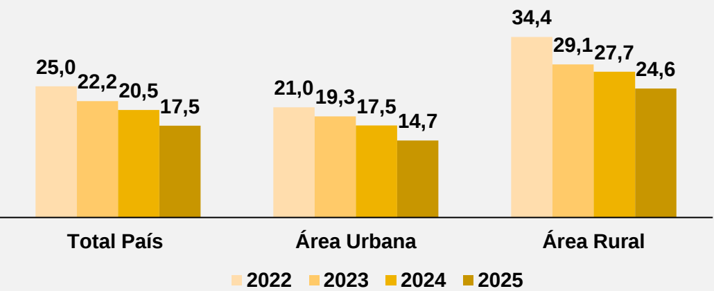
Factor de expansión revisión 2025
