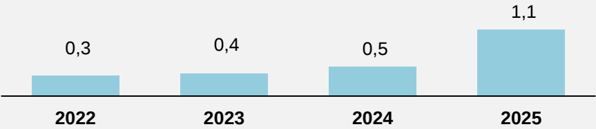
Área Rural. Método ajustado - método anterior
